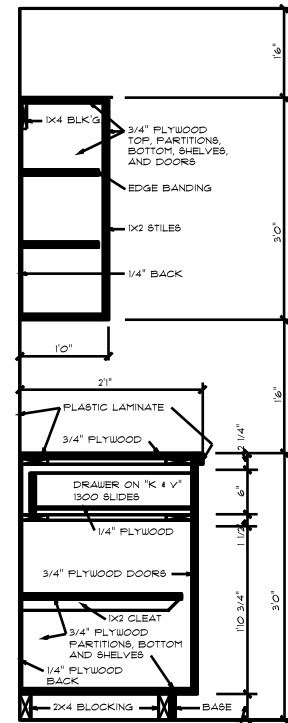
CABINET SECTION SCALE: 1" = 1'-0"
