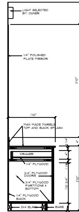
VANITY SECTION SCALE: 1" = 1'-0"
